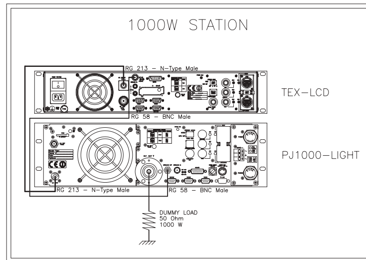
Figura 5.1: connessioni con l'amplificatore
