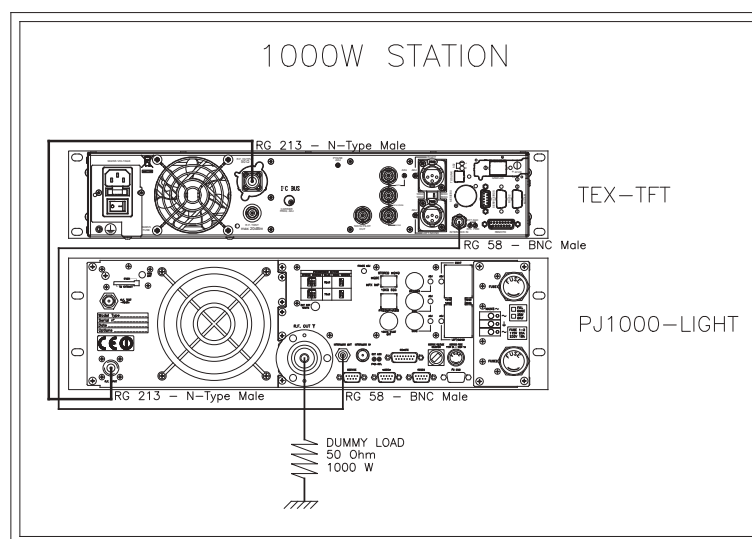
Figura 5.1: connessioni con l'amplificatore
