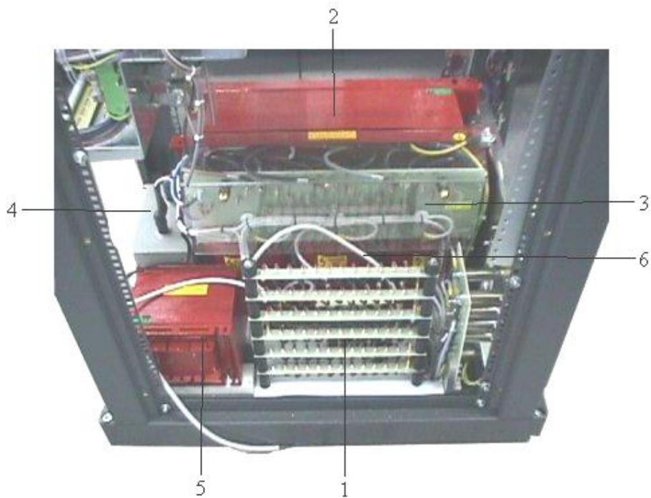
FIGURA 7 VISTA SEZIONE ALIMENTATORE P1
