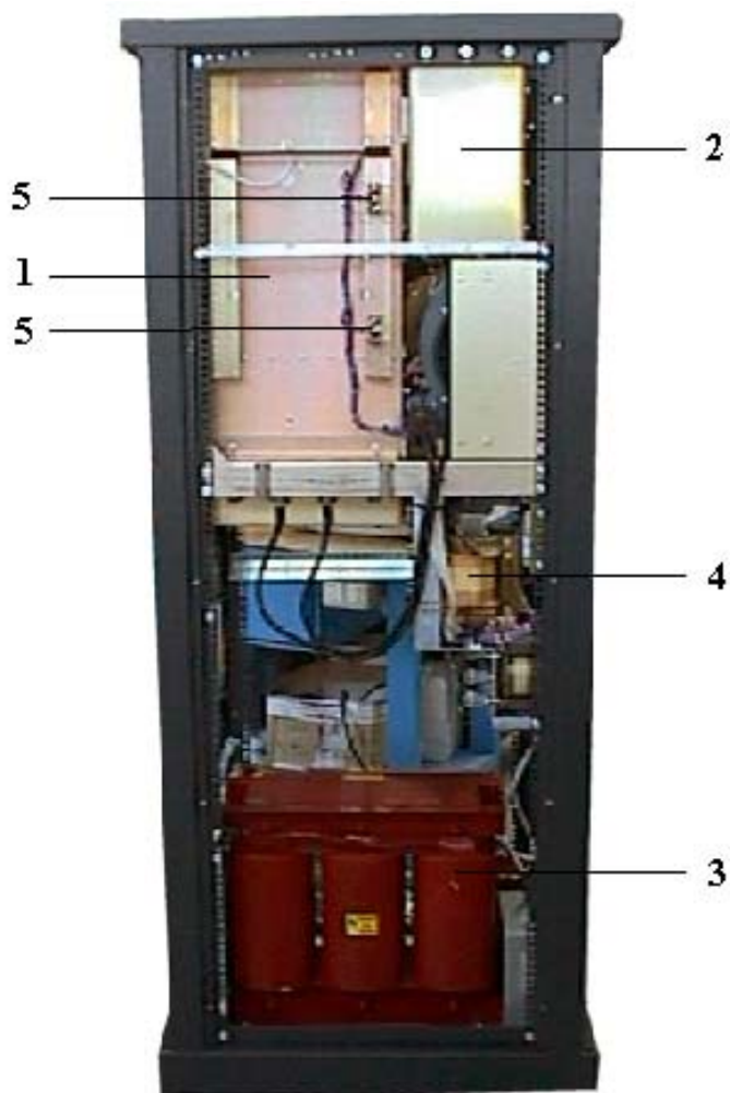
VISTA LATERALE CAMERA DESTRA RF
