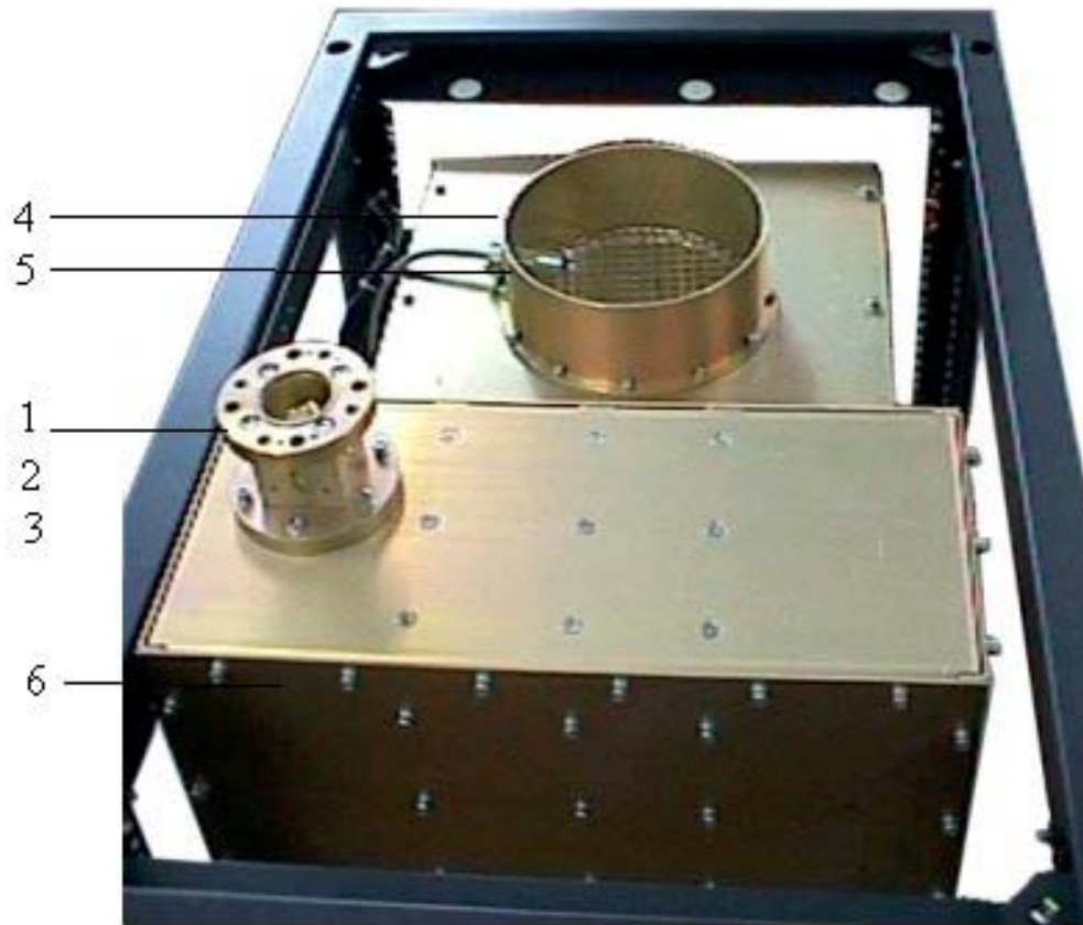
FIGURA 12 VISTA SUPERIORE CAMERA RF
