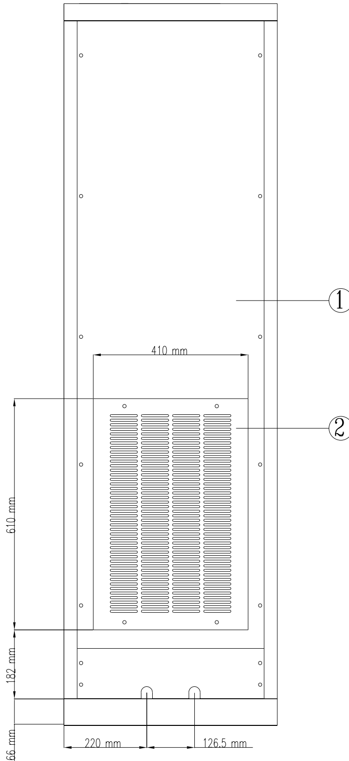
FIGURA 2 VISTA POSTERIORE
