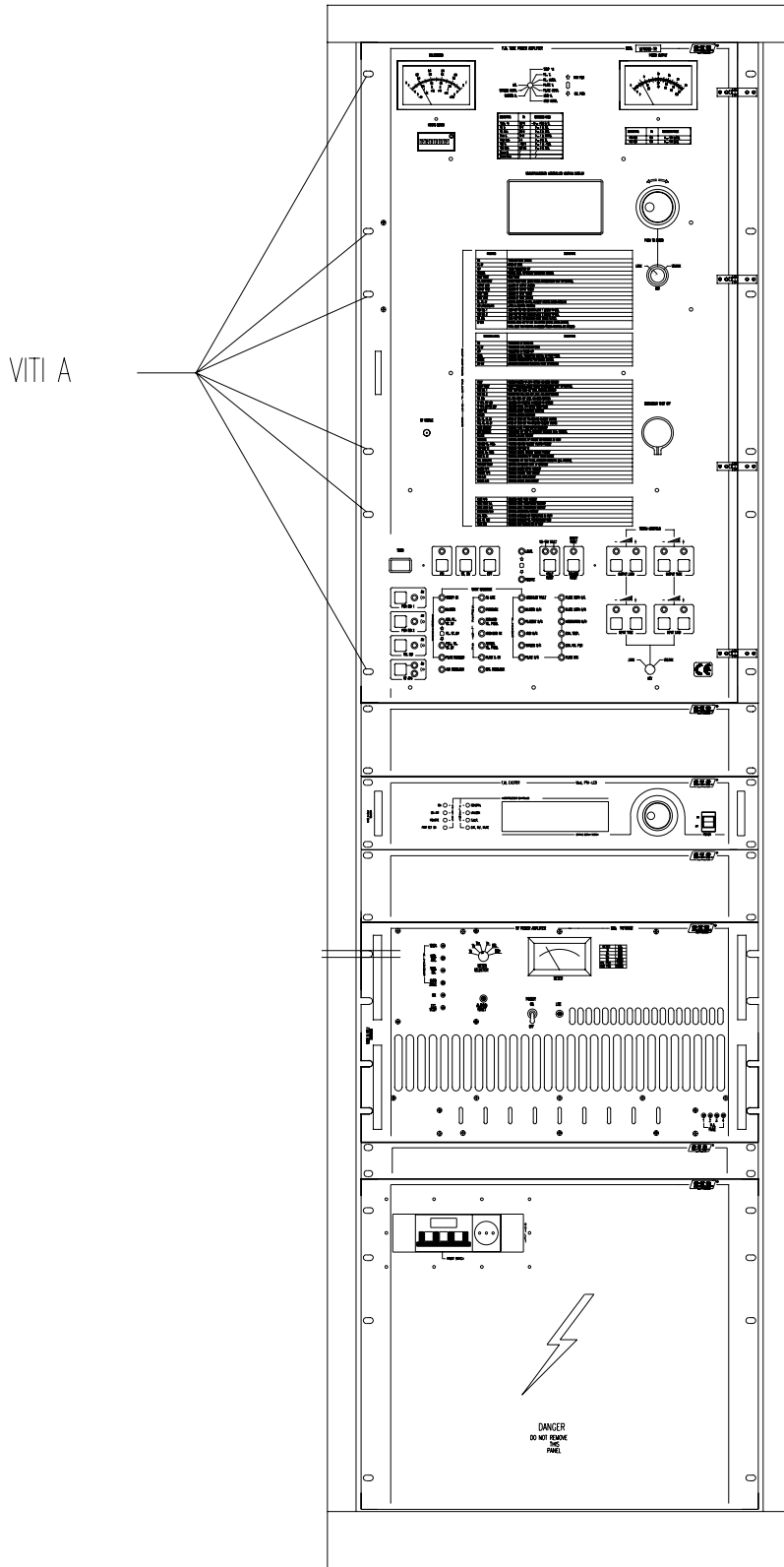
FIGURA 16 DIAGRAMMA INSTALLAZIONE VALVOLA N°1
