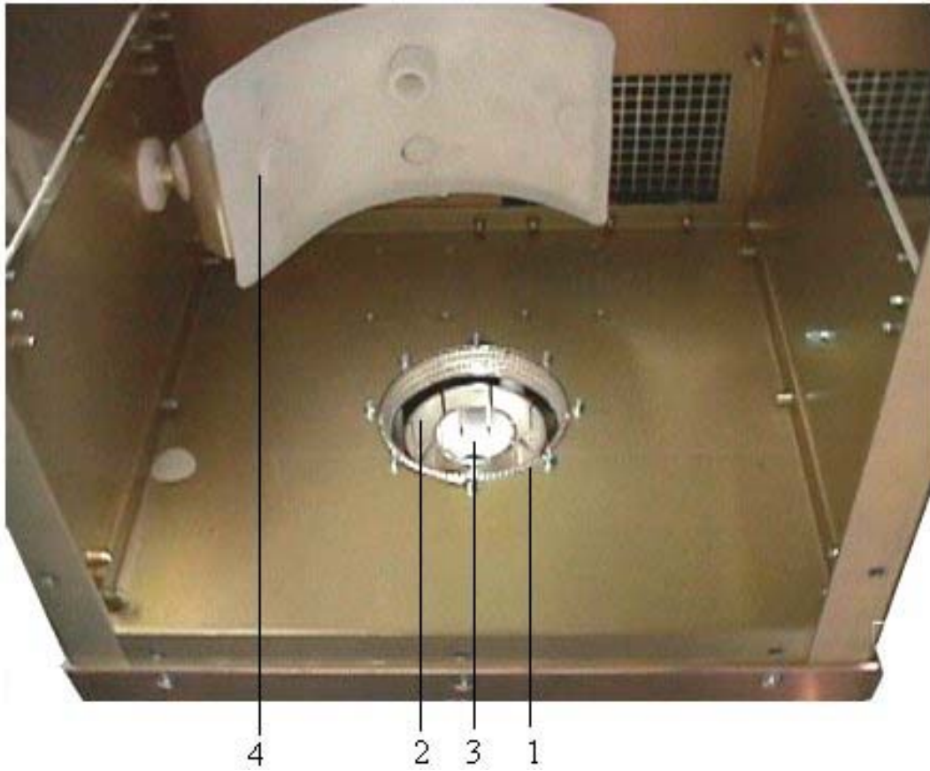
FIGURA 10 VISTA DELLO ZOCCOLO CAMERA RF
