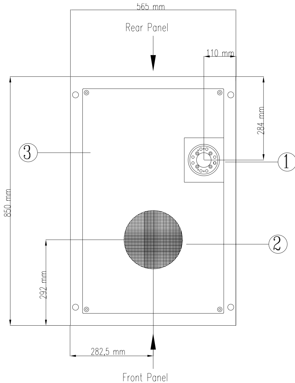
FIGURA 3 VISTA SUPERIORE
