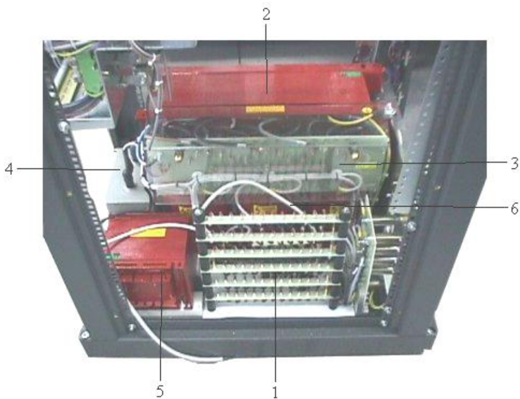
FIGURA 7 VISTA SEZIONE ALIMENTATORE P1
