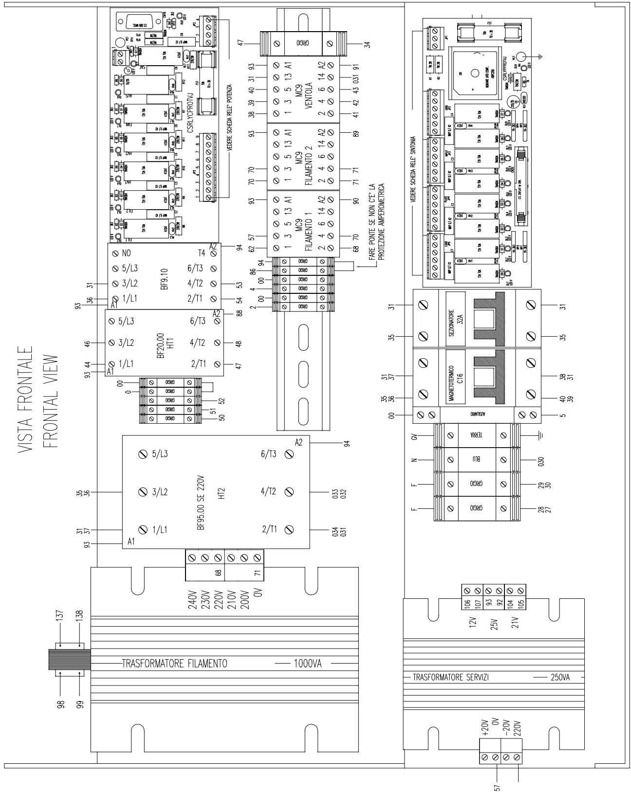
FIGURA 33 PIANO ELETTROMECCANICO (TRIODO)
