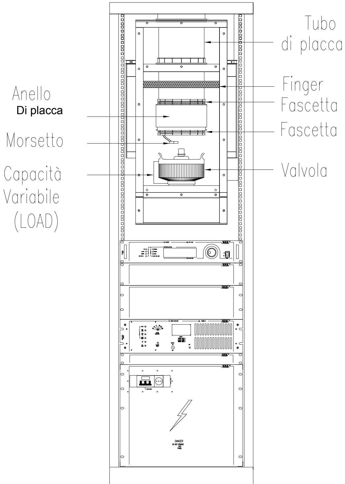
FIGURA 19 DIAGRAMMA INSTALLAZIONE VALVOLA N°3
