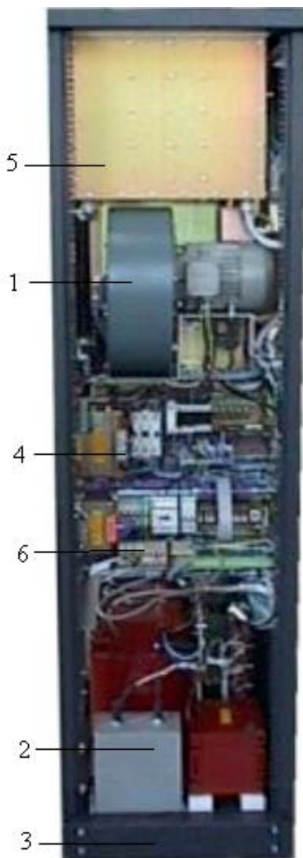
FIGURA 15 VISTA POSTERIORE
