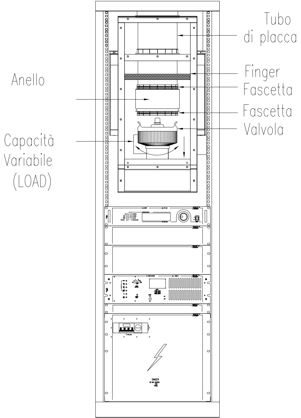
FIGURA 17 DIAGRAMMA INSTALLAZIONE VALVOLA N°2
