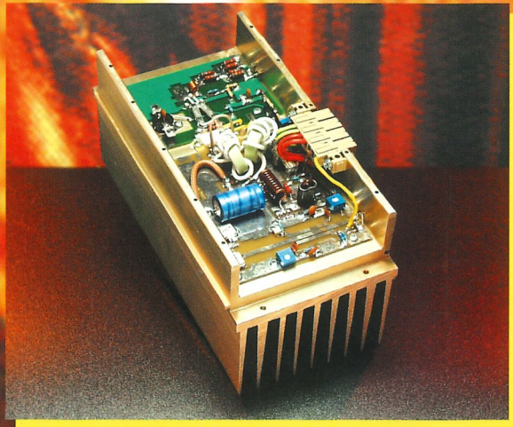
R.F. Module
