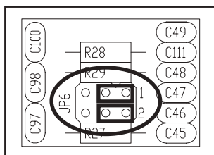
Ingressi Analogici
