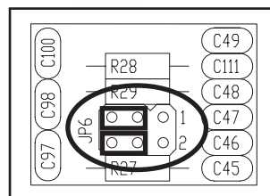
Ingressi I2C
